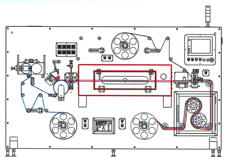
ソルベント塗工
