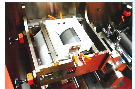
シップ薬塗工ヘッド (ダブルロール式)
